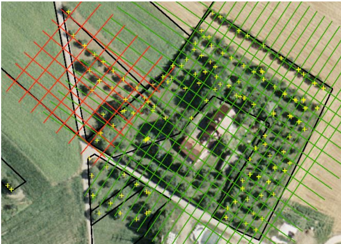
Abbildung 5: Vergleich des für das jeweilige Flurstück berechneten Pflanzrasters (rotes und grünes Gitter) mit den aus dem nDOM berechneten Stammstandorten (gelbe Kreuze). Im Hintergrund ist das entsprechende Ortho-Luftbild dargestellt (Quelle: eigene Darstellung, Luftbild: LGL Baden-Württemberg)
