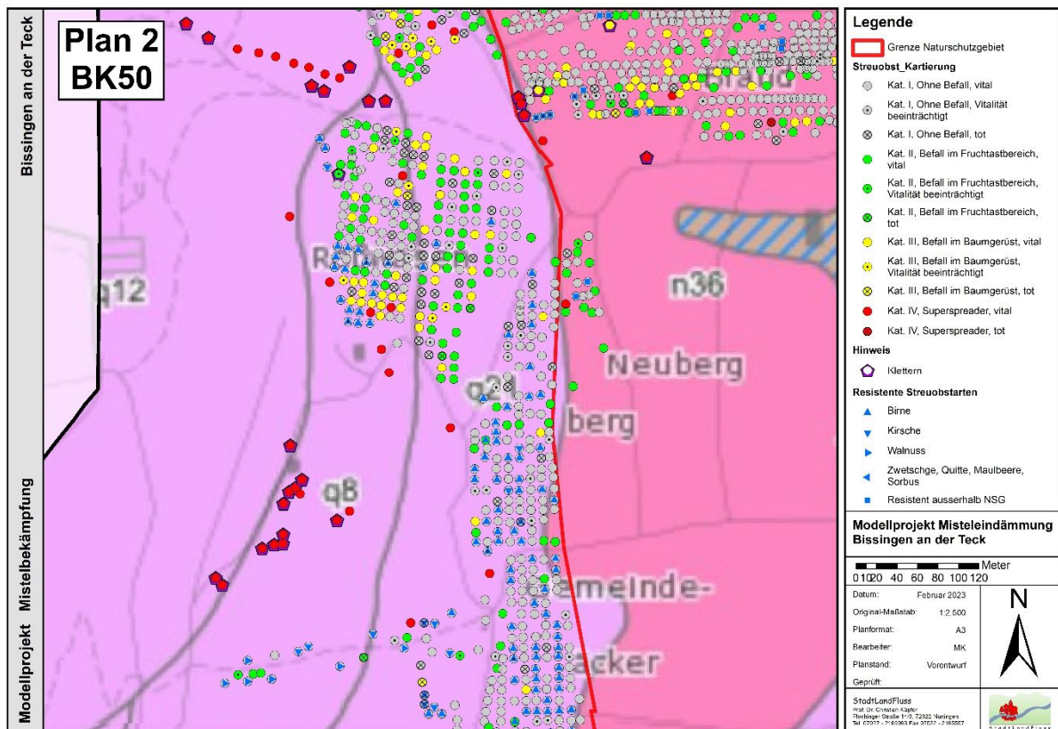
Abbildung 8: Bodenkundliche Einheiten zu Plan 2
